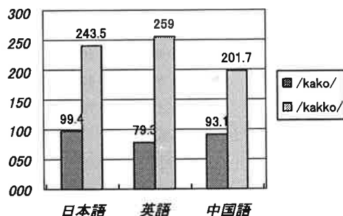
Figure 2 /kako//kakko/ 閉鎖区間長
