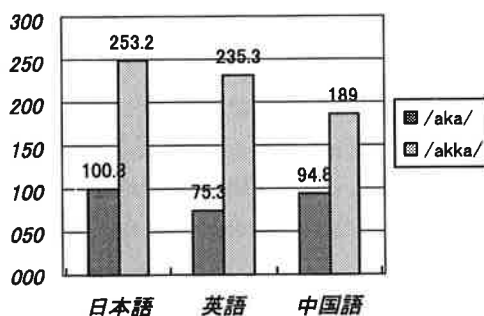
Figure 1 /aka//akka/の閉鎖区間長
